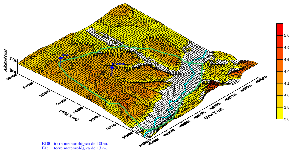
PLANTA DE ENSAYO DE AEROGENERADORES (CEDER) CAMPO DE VIENTO (4 x 3.5 Km) A 30 m a.g.l. MODELO WASP
